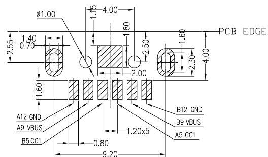
PCB LAYOUT 图仅供参考
