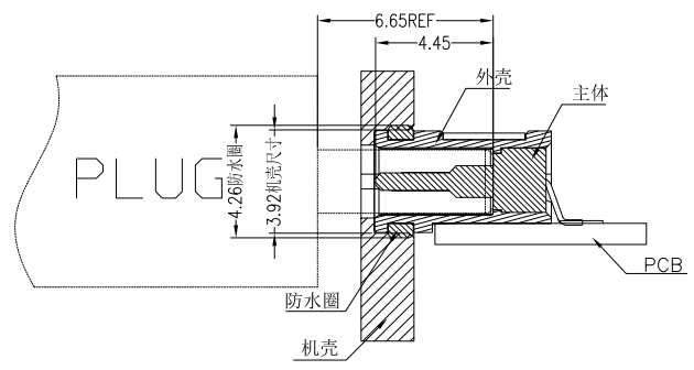
产品防水机构示意图
